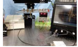
汎用超音波スキャナ (超音波顕微鏡モード)
