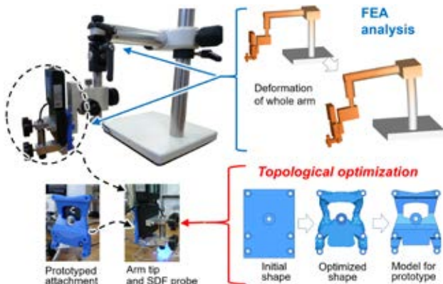
FEA及びボロロジー最適化を用いたSDF撮像用アーム型デバイス設計 Design of arm type device for SDF imaging by FEA and topological optimization
